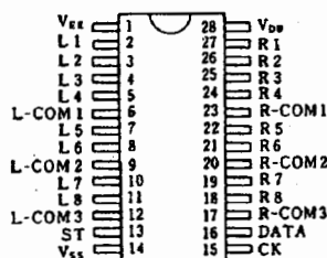
NJU7313AL
