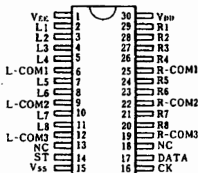
NJU7313AM
