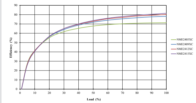
24V Inputs
