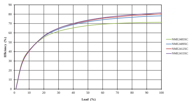
24V Inputs
