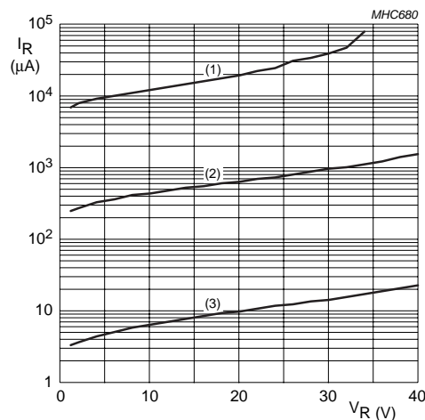
PMEG4010BEA/PMEG4010BEV
