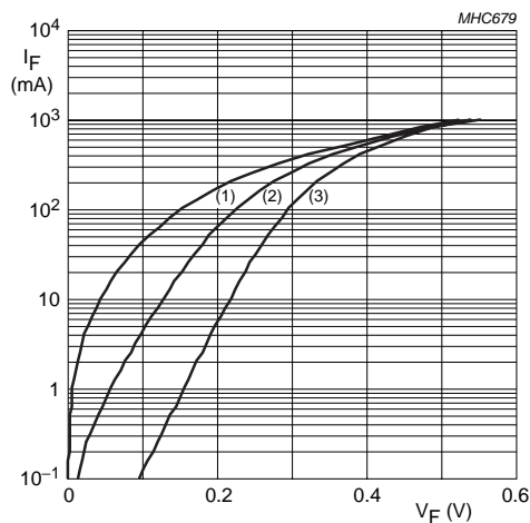
PMEG4010BEA/PMEG4010BEV
