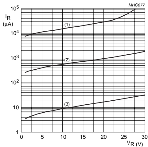
PMEG3010BEA/PMEG3010BEV
