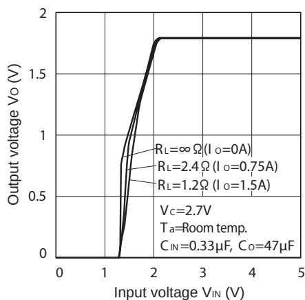
Fig.15 Output Voltage vs. Input Voltage (PQ018EZ1HZxH)
