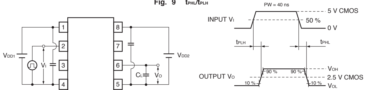
Fig. 9 t_{PHL}/t_{PLH}
