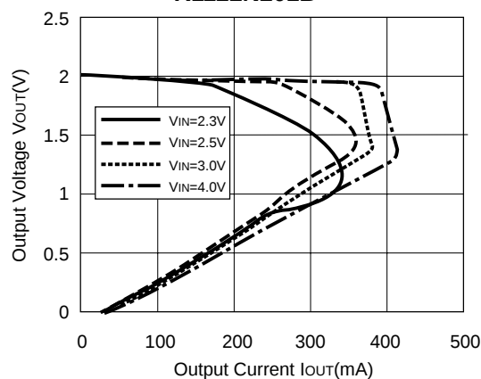
R1122N201B
