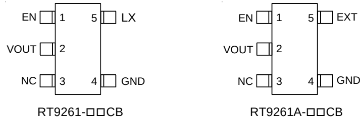
SOT-23-5
