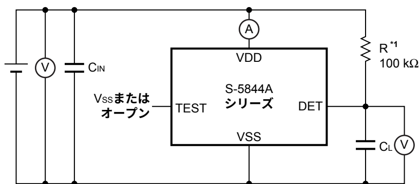
図6 測定回路1
