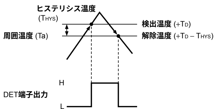
図10 DET端子出力論理がアクティブ "H" の場合の動作
