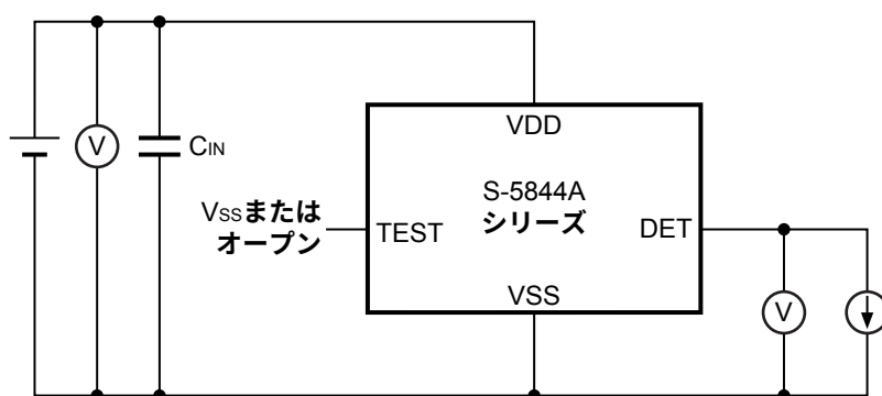
図7 測定回路2
