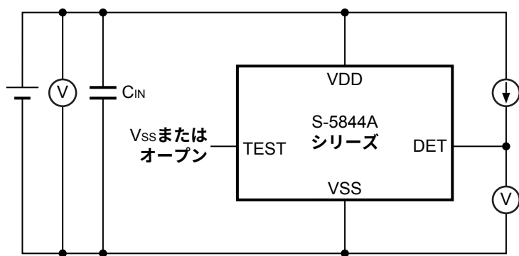
図8 測定回路3
