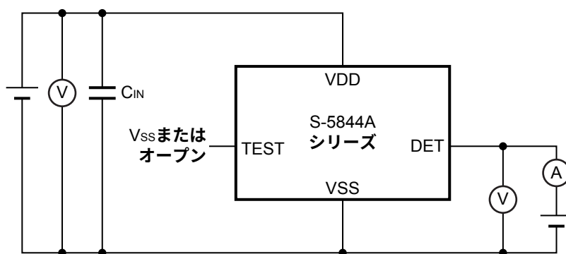
図9 測定回路4
