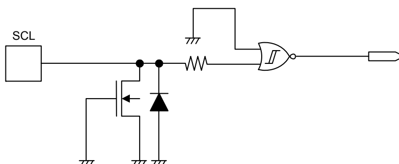
図7 SCL端子
