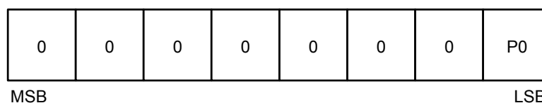
図 12 ポインタレジスタ構成
