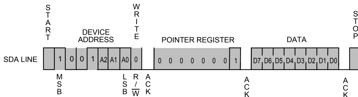
図 19 書き込み動作
