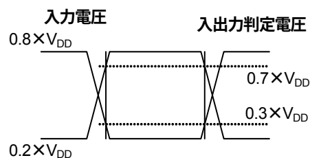
図 8 AC 測定入出力波形
