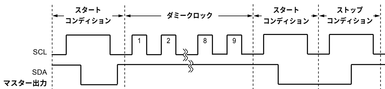
図 24 バスの解放方法
