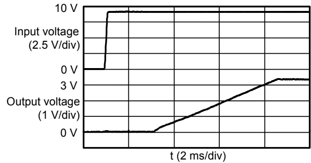
S-8533A50AFT ( V_{IN} : 0\text{ V} \rightarrow 9.0\text{ V} )
