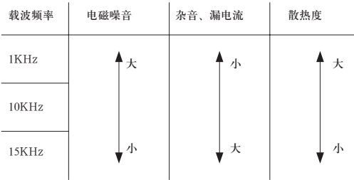
图4-2 载波频率对环境的影响关系图
