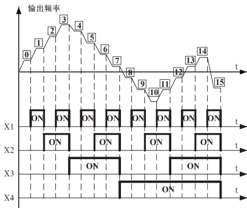
图4-25 多段速运行逻辑图
