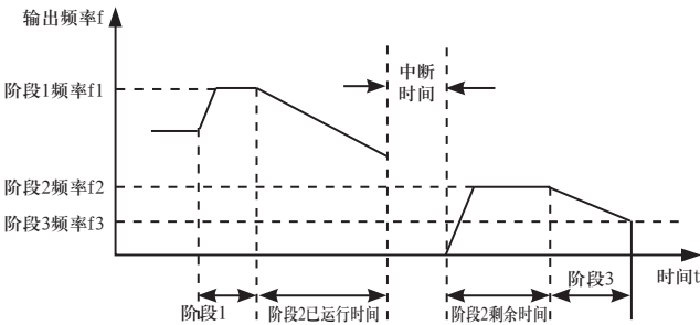
图4-26 简易PLC启动方式1
