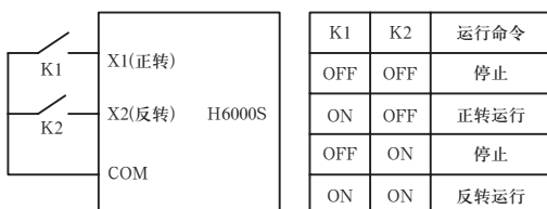
图4-7 两线式控制（运行与方向合一）
