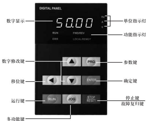
图3-1 操作面板示意图
