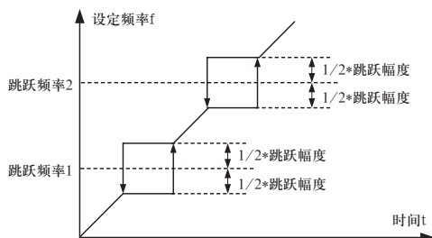
图4-16 跳跃频率示意图
