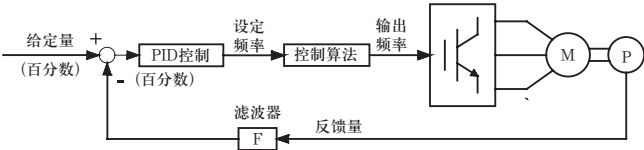
图4-22 过程PID原理框图
