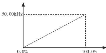
图4-13 给定量与高速脉冲量输出的对应关系
