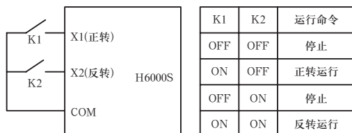
图4-8 两线式控制（运行与方向分离）
