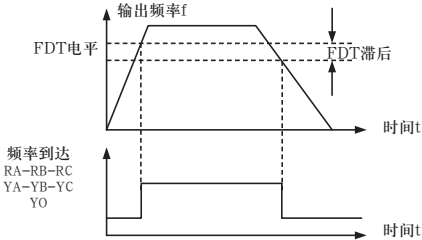
图4-19 FDT电平示意图
