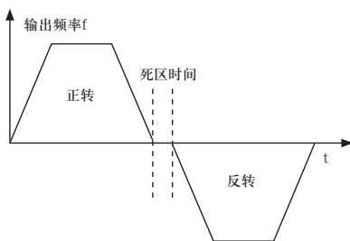
图4-15 正反转死区时间示意图
