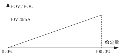
图4-12 给定量与模拟输出对应关系
