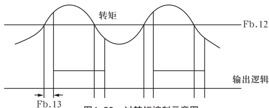
图4-30 过转矩控制示意图
