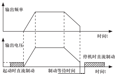
图4-14 直流制动示意图
