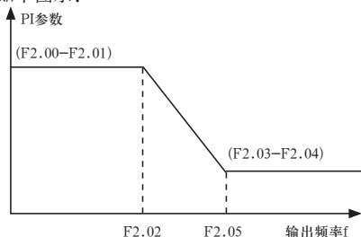
图4-3 PI参数示意图
