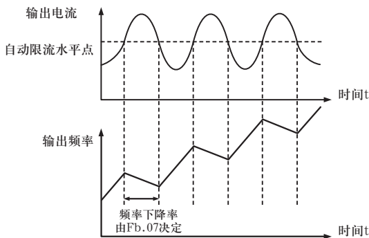
图4-29 限流保护功能示意图
