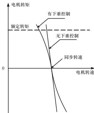
图4-21 下垂控制电机特性示意图
