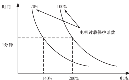
图4-27 电机过载保护系数设定
