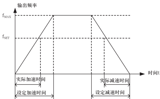
图4-1 加减速时间示意图
