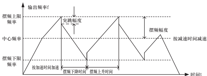
图4-17 摆频运行示意图
