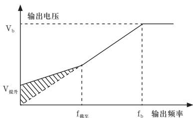
图4-5 手动转矩提升示意图
