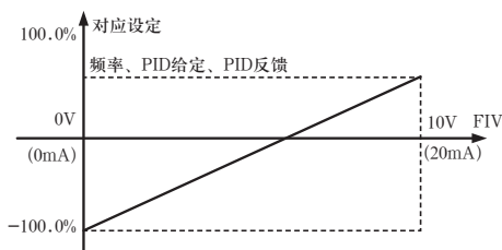
图4-11 模拟给定与设定量的对应关系
