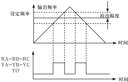
图4-20 频率到达检出幅值示意图
