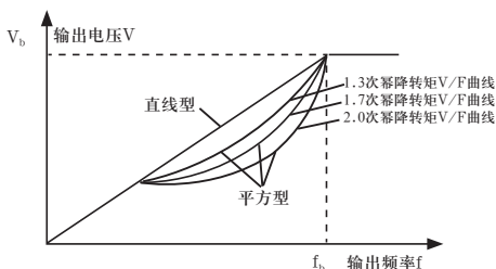
图4-4 V/F曲线示意图
