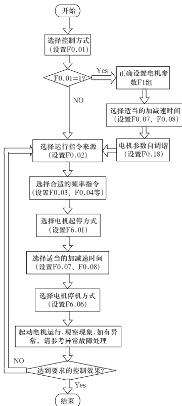
图3-3 快速调试流程图
