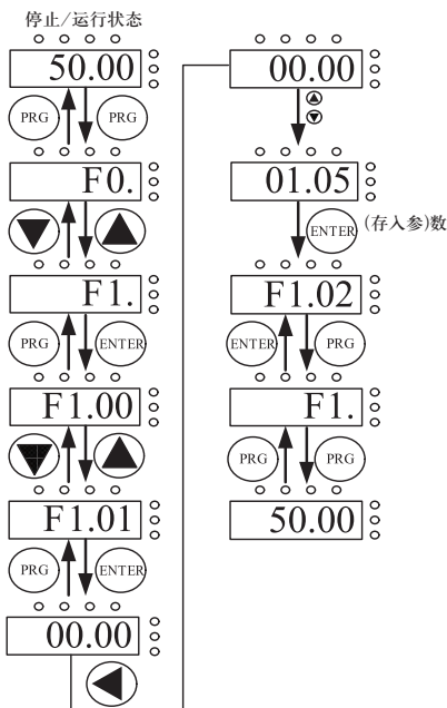
图3-2 三级菜单操作流程
