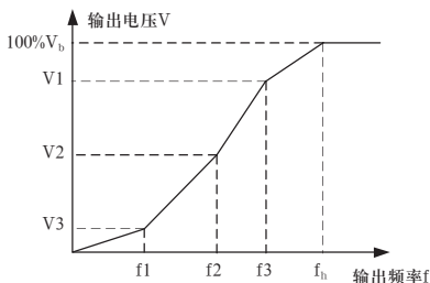
图4-6 V/F曲线设定示意图
