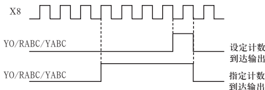
图4-18 设定计数值和指定计数值示意图
