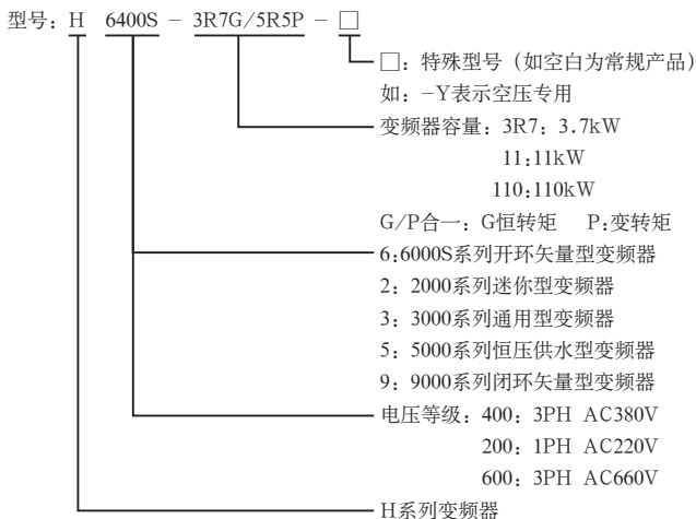
图1-1 变频器铭牌说明
