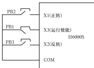
图4-10 三线式控制模式2
