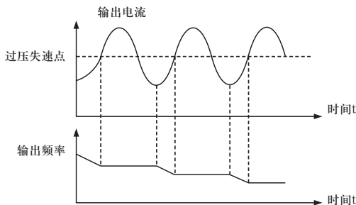
图4-28 过压失速功能
