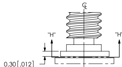
DETAIL 'G' SCALE 8 : 1
