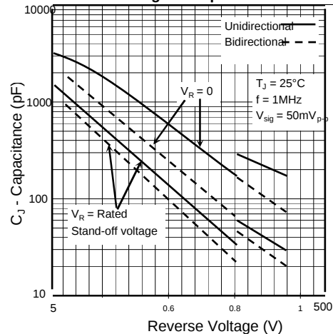
Fig. 6 - Capacitance
