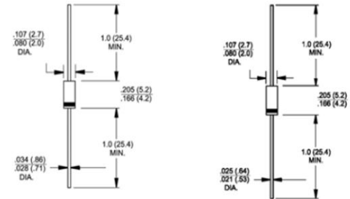
DO-204AL (DO-41)
