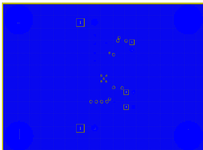
(IN2 layer)
