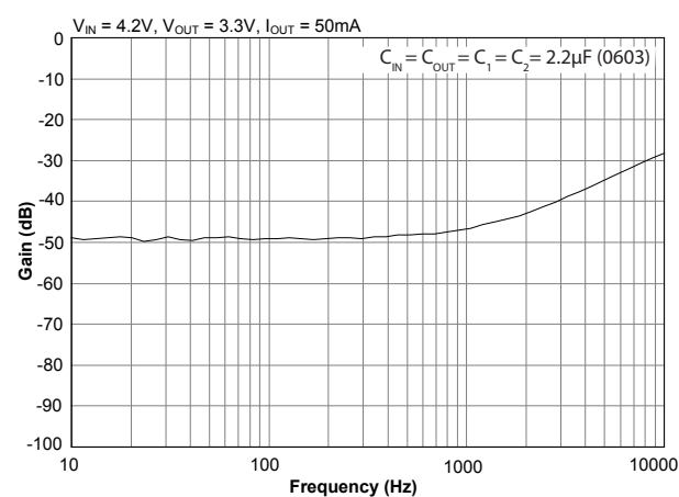
PSRR — 1x Mode
