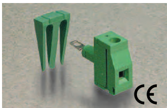
MPT-275/ CMR-75
