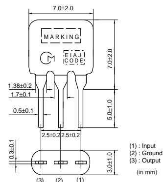
SFELF10M7FA0G-B0
