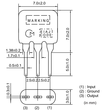
SFELF10M7FA00-B0
