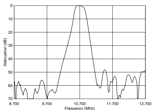
SFELF10M7FA00-B0
