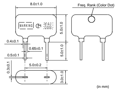
CDALF10M7G_Series
