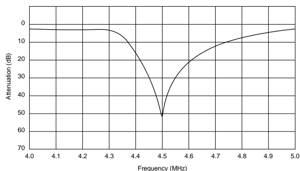
TPSKA4M50B00-R1
