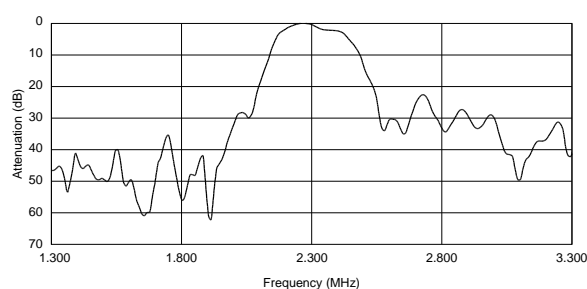
SFSKB2M30GF00-R1
