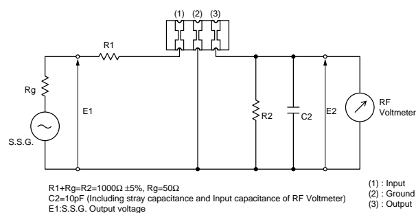
SFSKA4M50CF00-R1
