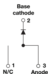
TO-263AB (D²PAK)
