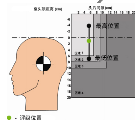
图5 头枕评级（高度调节可锁止，倾斜调节无锁止）
