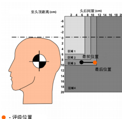
图4 头枕评级（倾斜可调节不可锁止）
