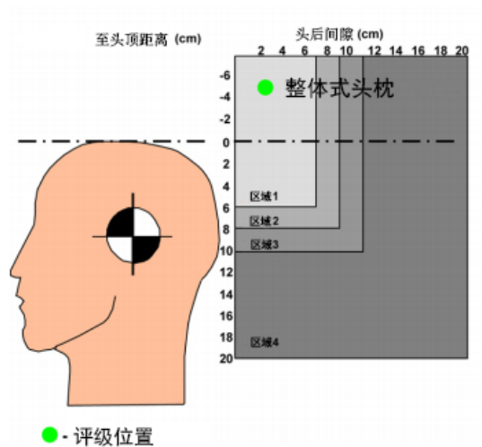
图2 头枕评级（整体式/固定式）
