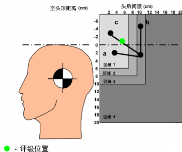
图7 头枕评级（高调和倾斜调节均可锁止）
