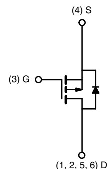
P-Channel MOSFET
