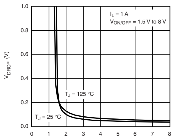
V_{IN} (V)
