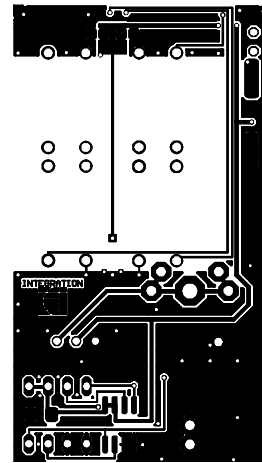
Bottom Layer
