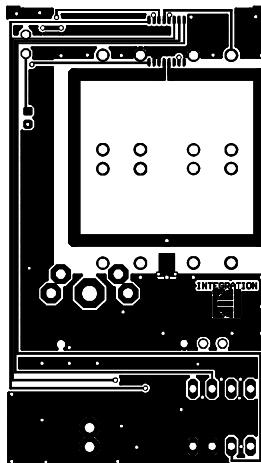
Top Layer
