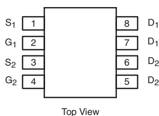
SO-8
