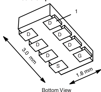
1206-8 ChipFET ®
