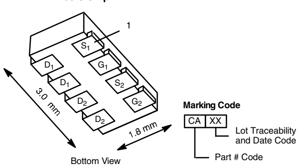
1206-8 ChipFET®
