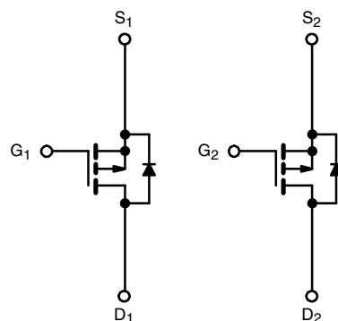
P-Channel MOSFET
