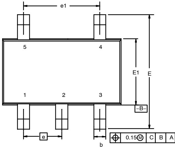
SOT23-5L Format
