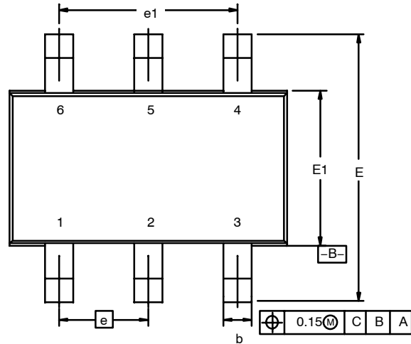
SOT23-6L Format
