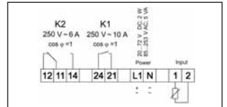
Abb. 3: Anschlussschema Fig. 3: Connection diagram Fig. 3: Schema de connexion Afb. 3: Aanslutingschema Bild 3: Anslutningsschema Fig. 3: Schema d'allacciamento Imagen 3: Esquema de conexión 図 3: 結線図
