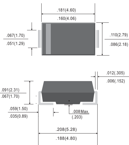
SMA(DO-214AC)
