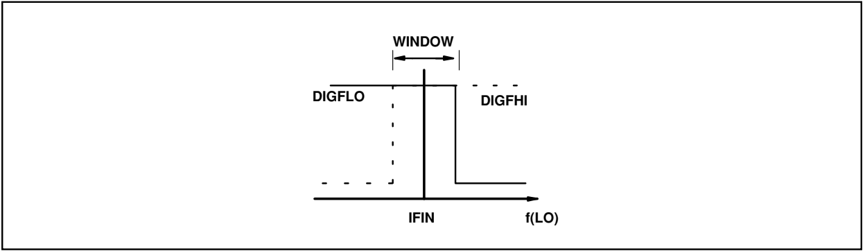
Fig. 7 SL1466 digital AFC output
