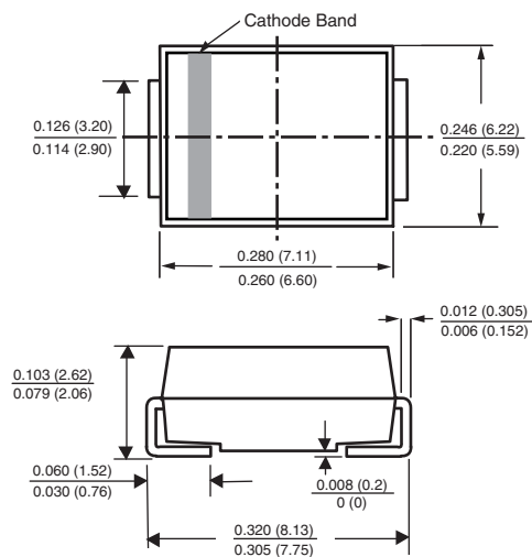
DO-214AB (SMC J-Bend)
