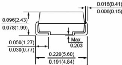
SMA/DO-214AC
