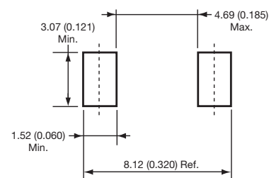
DO-214AB (SMC)
