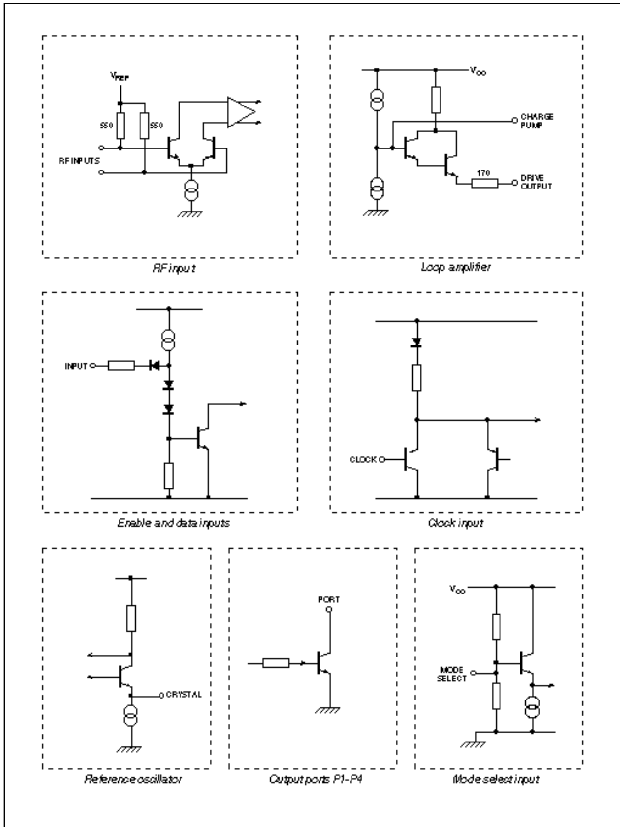
Fig. 7 SP5054 input/output interface circuits
