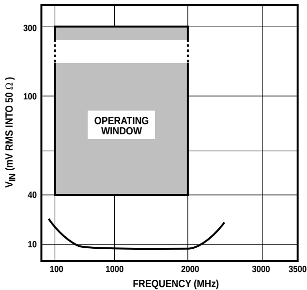
Figure 4a - Prescaler disabled, PE = 0
