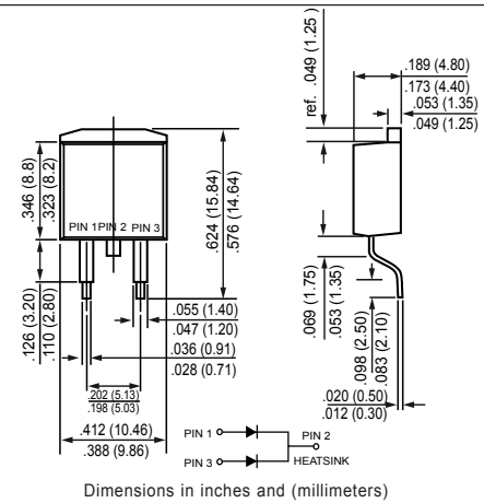
D2-PAK
