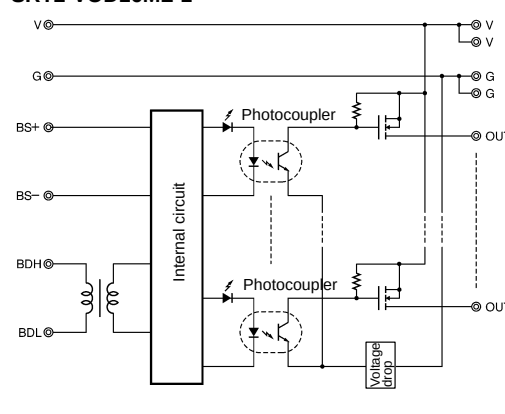
SRT2-VOD16ML-1
