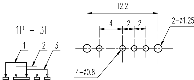
示意图 SCHEMATIC
