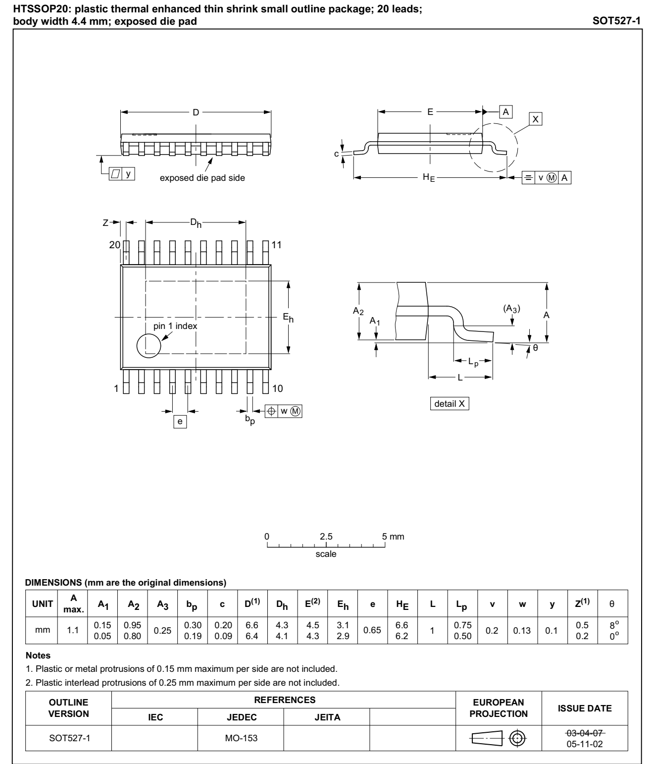
Fig 8. SOT527-1 (HTSSOP20)
