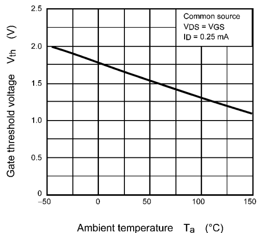
Fig. 7.6 V_{th} - T_a
