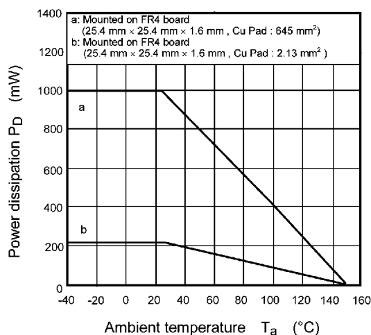
Fig. 7.14 P_D - T_a
