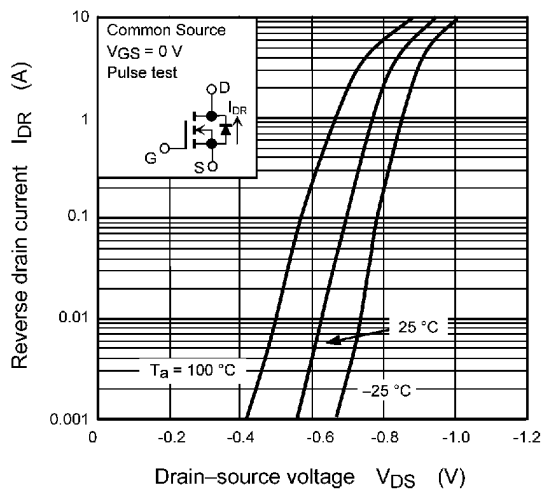
Fig. 7.9 I_{DR} - V_{DS}
