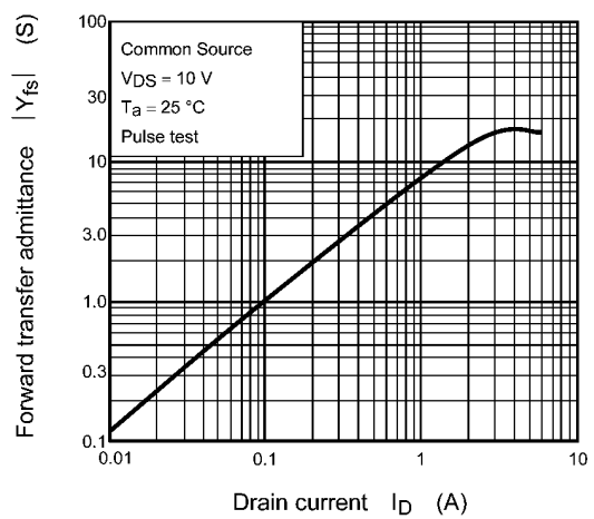
Fig. 7.8 |Y_{fs}| - I_D
