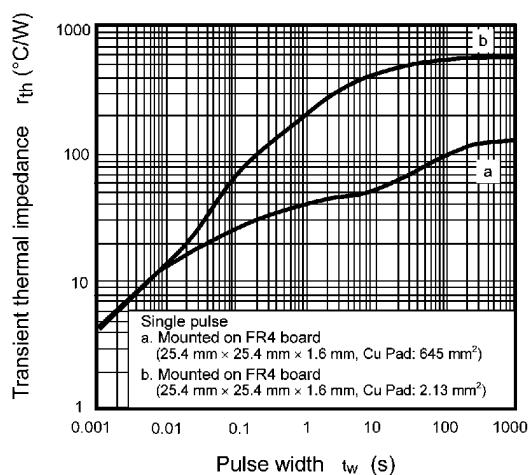
Fig. 7.13 r_{th} - t_w
