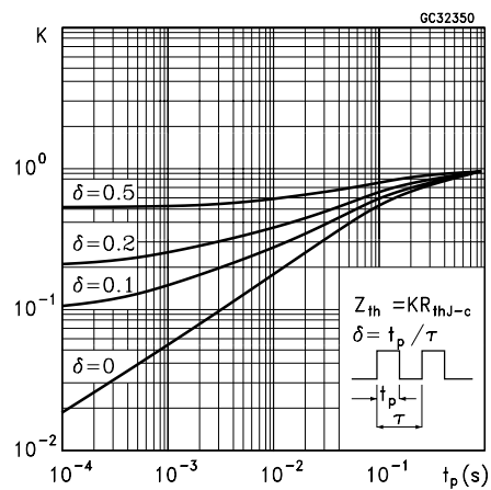
Thermal Impedance
