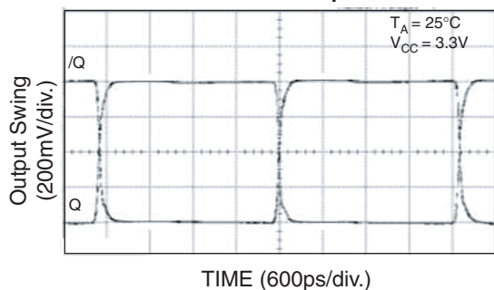
200MHz Output
