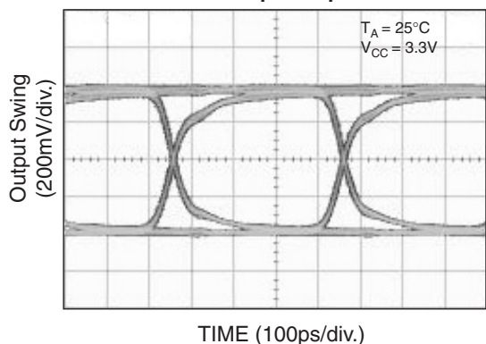
2.5Gbps Output
