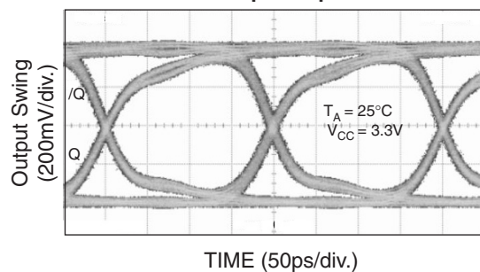
5Gbps Output
