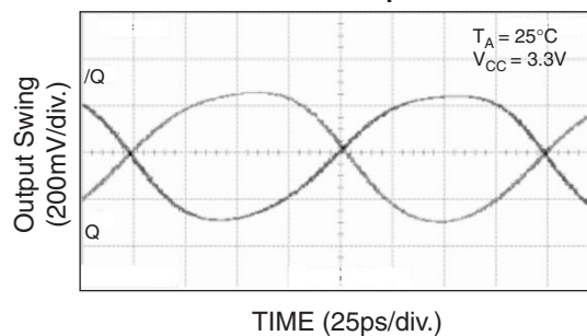
5GHz Output
