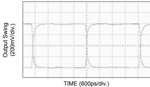
200MHz Output
