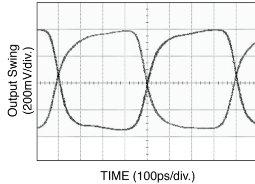
1.25GHz Clock
