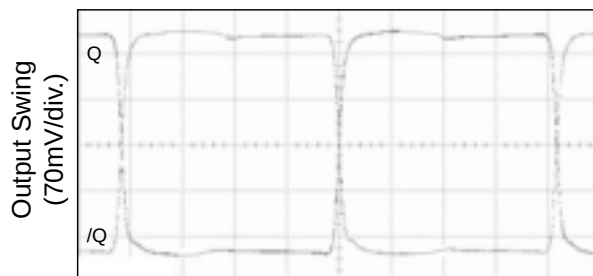
200MHz Output
