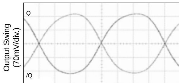
2.5GHz Output
