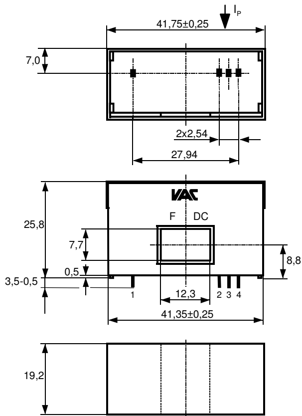
Maßbild Nr. 1
