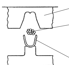
Obermatrize (Crimpstempel)
