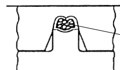
Die geschrägten Außenflanken dienen der besseren Führung der Crimphülse in der Obermatrize als auch dem besseren Einrollen der Crimphülsenflanken
