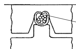
Die beiden eingerollten Crimphülsenflanken treffen sich in der Obermatrize und werden nach innen gepresst
