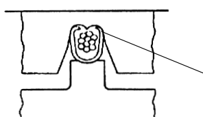
Obermatrize und die sich einrollenden Crimphülsenflanken zwingen das abisolierte Leiterende in den Crimphülsenboden
