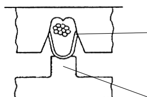
Die geschrägten Außenflanken dienen der besseren Führung der Crimphülse in der Obermatrize als auch dem besseren Einrollen der Crimphülsenflanken
